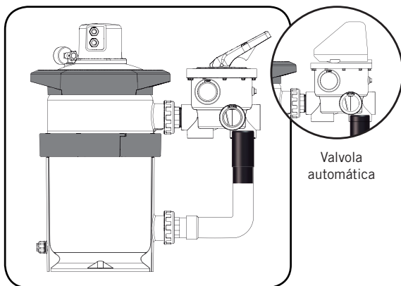
- Incollare manicotto 65289 -
