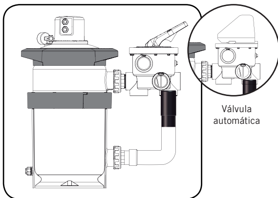
- Encaixar manga 65289 -
