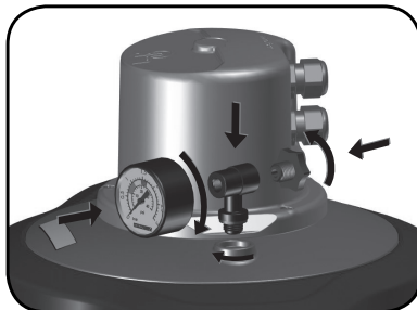
- Montage des Manometers -
