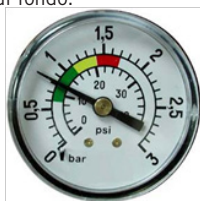
0,8 kg/cm 2 : Pressione iniziale di un filtro all'inizio di un ciclo di filtraggio
