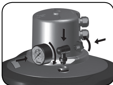
- Montagem manômetro -
