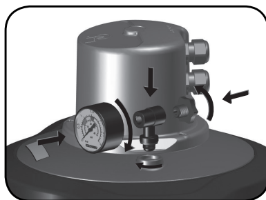
- Montaggio manometro -
