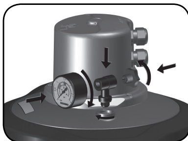
- Montaje manómetro -
