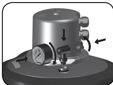
- Montage du manomètre -
