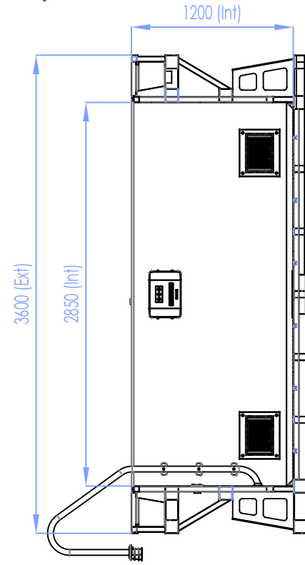
A-A
