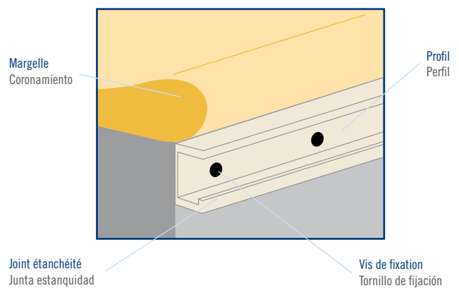
Fixation type “HUNG” pour rénovations Hung type fastening for renovations
