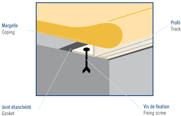
Fixation type “HUNG” pour piscines à construire Hung type fastening for pools to be built
