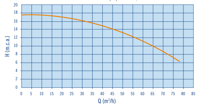
Equipo contracorriente Eco 4,5 CV III Eco countercurrent equipment 4,5 CV III
