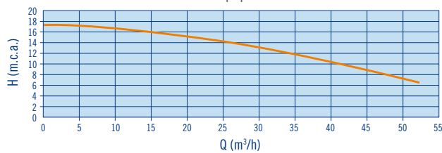
Equipo contracorriente Eco 3 CV II - 3 CV III Eco countercurrent equipment 3 CV II - 3 CV III
