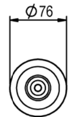
Flotador Mod. 92
