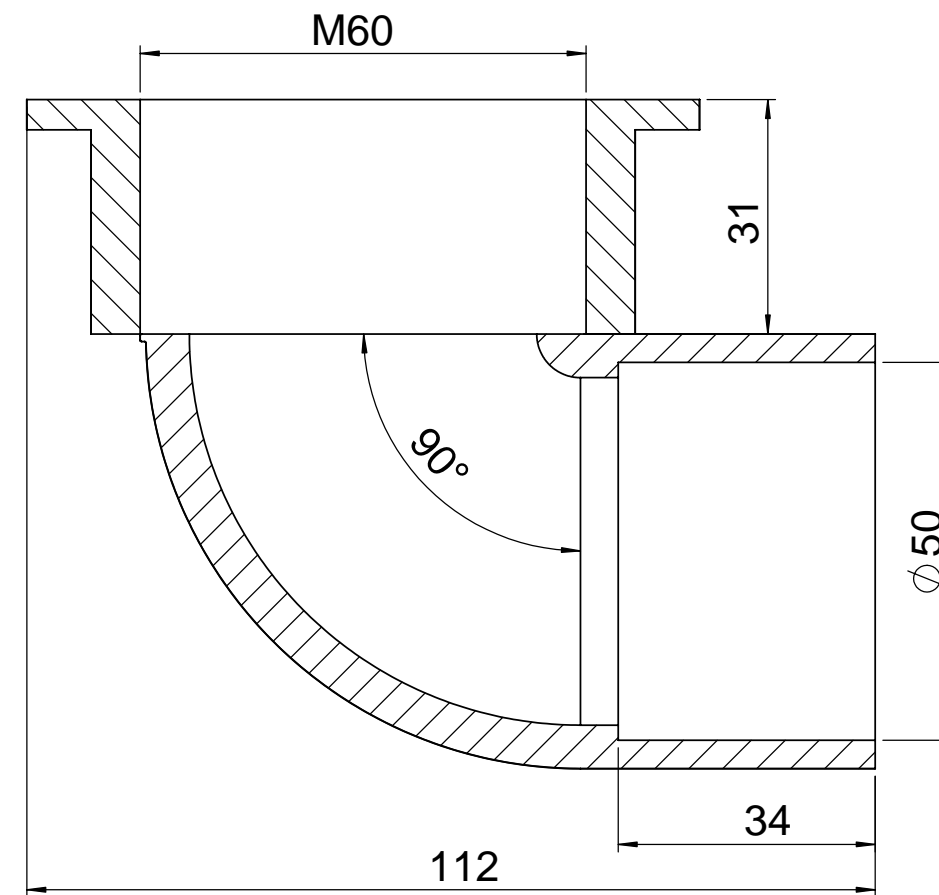
SECCIÓN A-A ESCALA 1 : 1
