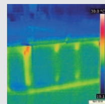
Verifica delle perdite di calore nel Nordic Insulation System
