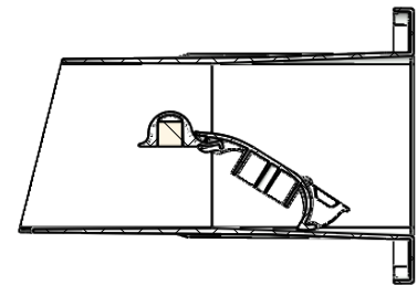
SECCIÓN A-A
