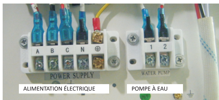
380 - 400V / 3ph / 50Hz
