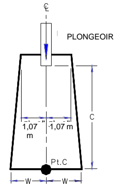
ZONE DE DÉGAGEMENT MINIMALE D'UN PLONGEOIR
